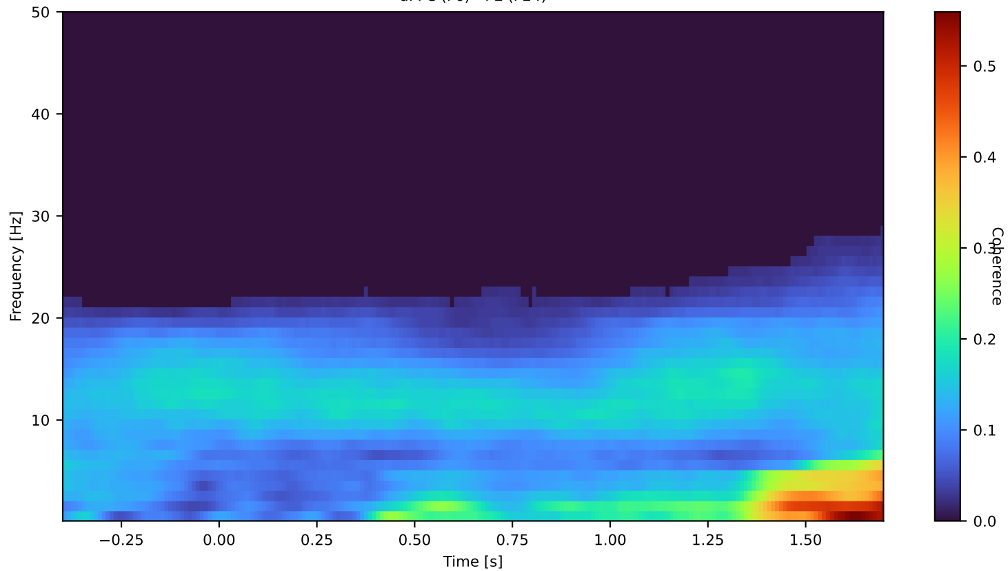
dPFC (F6) - PE (P24)
